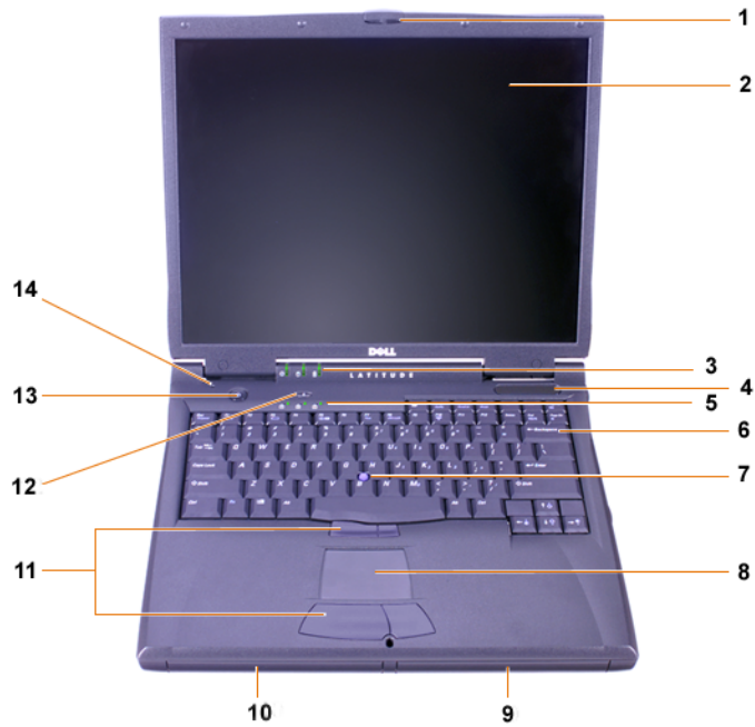
图 2-4: 正面视图
